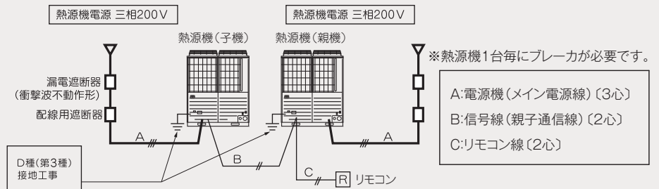
(i) 配線系統図
