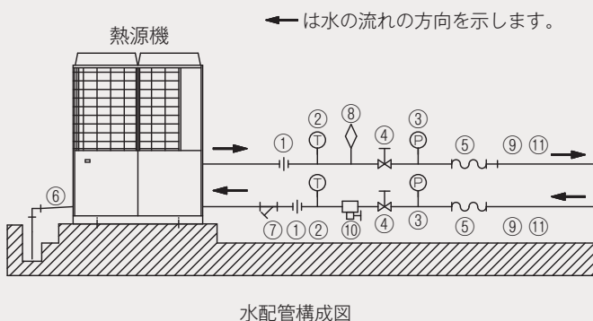
水配管構成図
